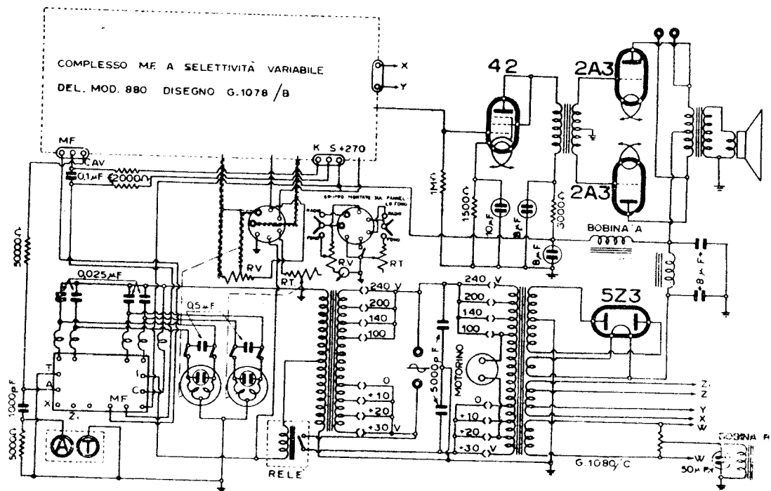
F.I.M.I. - MOD. PHONOLA « 910 » - PARTE BF
