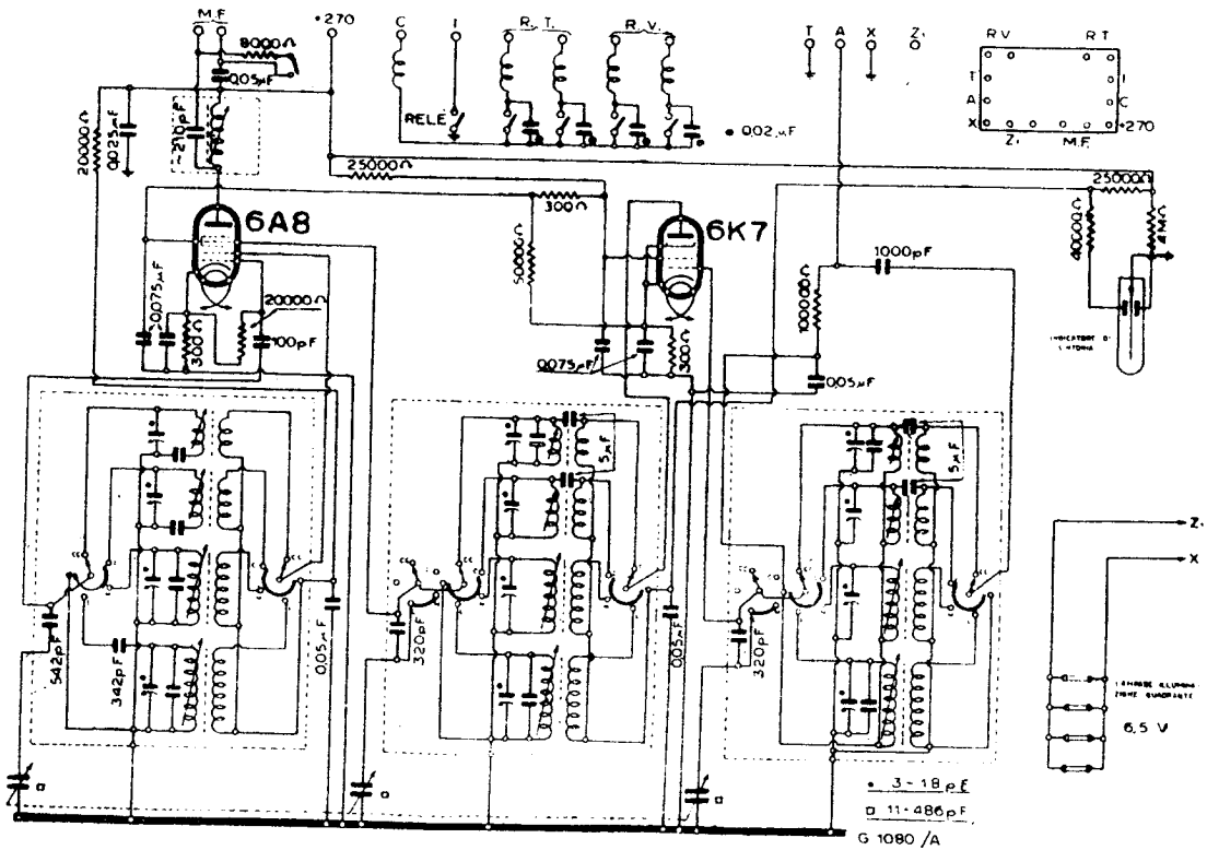
F.I.M.I. - MOD. PHONOLA « 910 » - PARTE AF (MF DELL'« 880 »)
